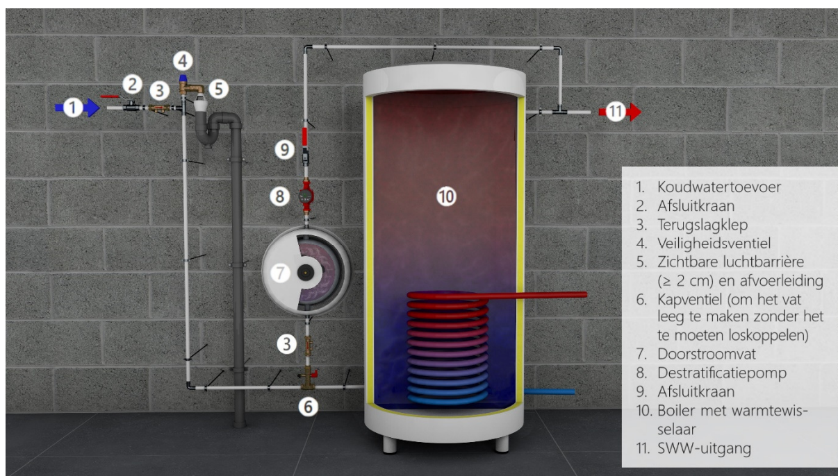
Figuur 1: boiler met destratificatiepomp en doorstroom expansievat
